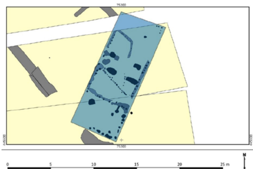
Plattegrond van het drieschepige huis (Transect).
