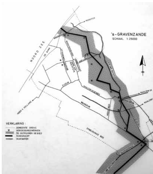
Tracé van de tankgracht en het daarbij behorende schootsveld. Collectie Jan Dahmeijer.
